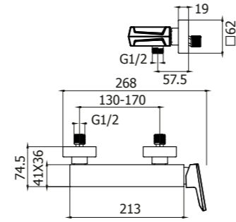
Miscelatore doccia senza kit doccia. Single-lever shower mixer without shower kit.
