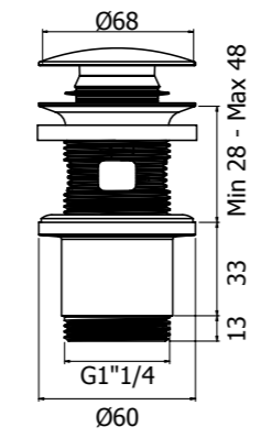
Piletta di scarico click-clack in acciaio inox, con troppo pieno Click-clack waste slotted, stainless steel
