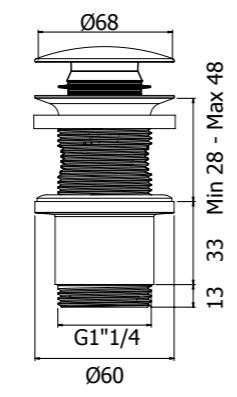
Piletta di scarico click-clack in acciaio inox, senza troppo pieno Click-clack waste unslotted, stainless steel
