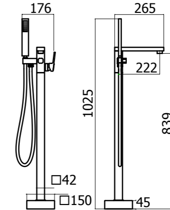
Miscelatore vasca a pavimento con kit doccia. Kit di fissaggio venduto separatamente
